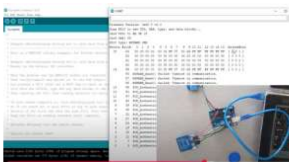
Gambar 6. Proses Pemrograman
