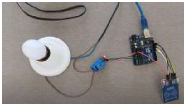
Gambar 7. Proses Pemograman
